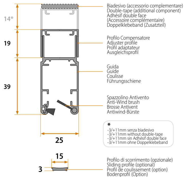
Sezione verticale - Vertical section Section verticale - Vertikaler Schnitt
